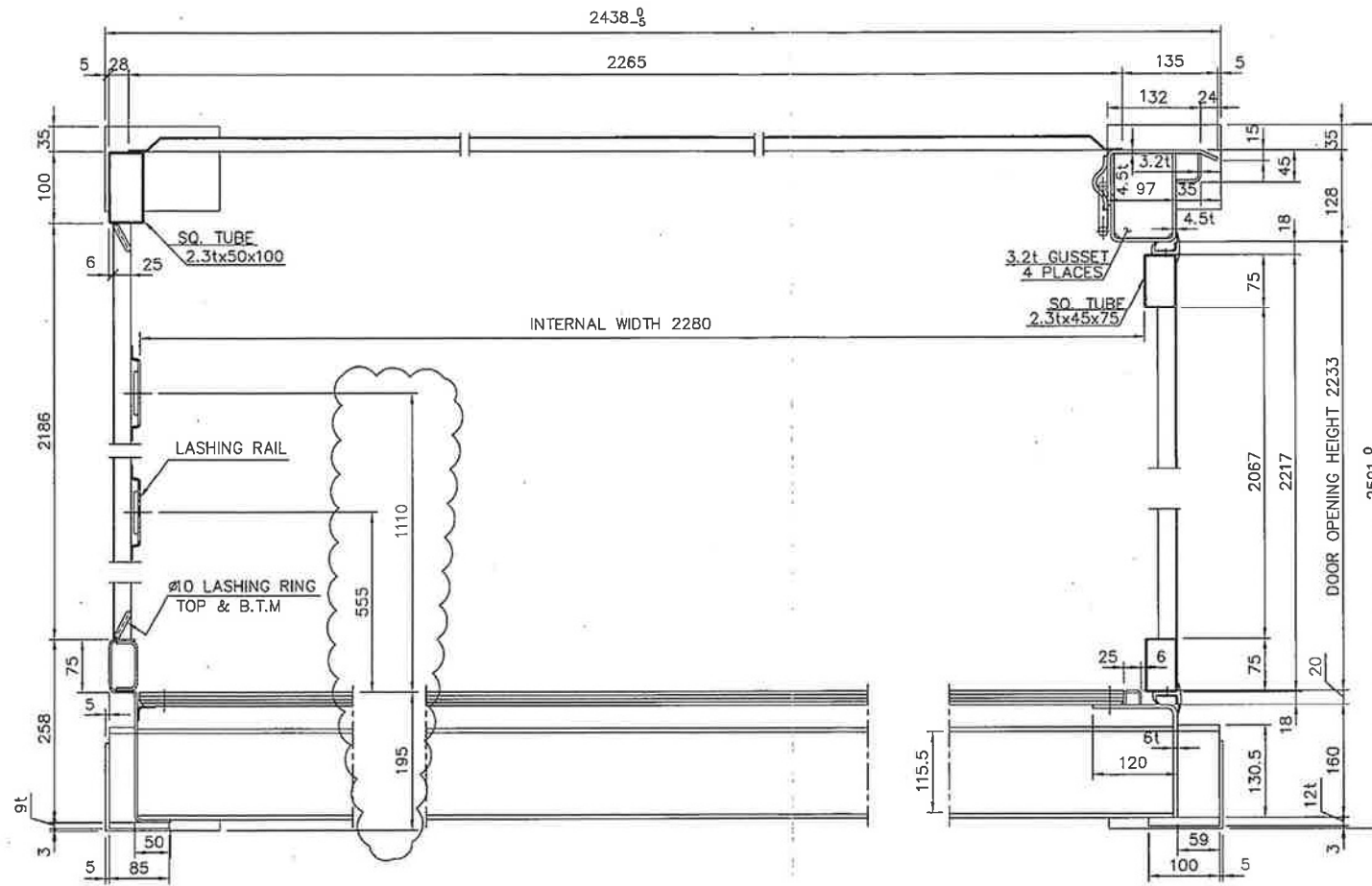
SECTION A-A
