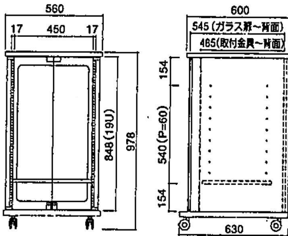
機器収納ラック (共栄商事製 EIA-970DX)
