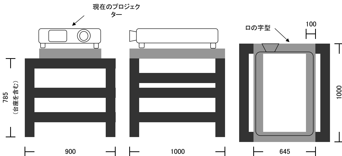
プロジェクター設置台 (特型スチール製)
